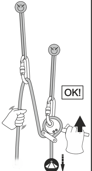
Рис. 7б. Спуск груза
