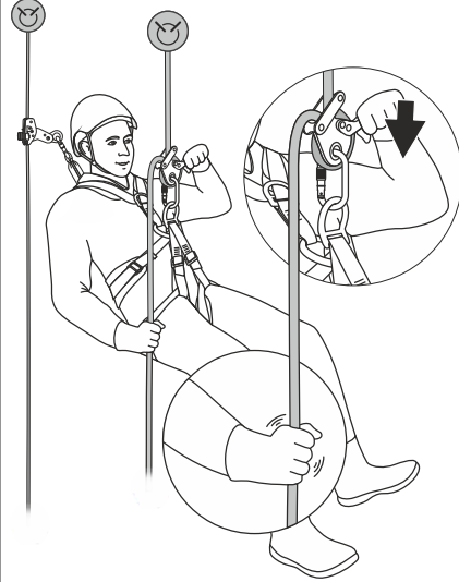
Рис. 8. Подъем с использованием зажима со стремнем
