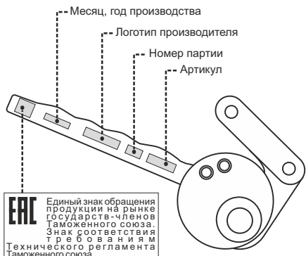
Рис. 1. Состав, идентификация и маркировка изделия
