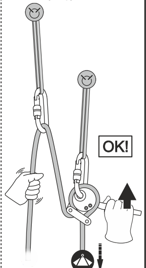
Рис. 7б. Спуск груза
