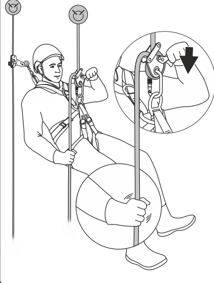
Рис. 8. Подъем с использованием зажима со стремнем
