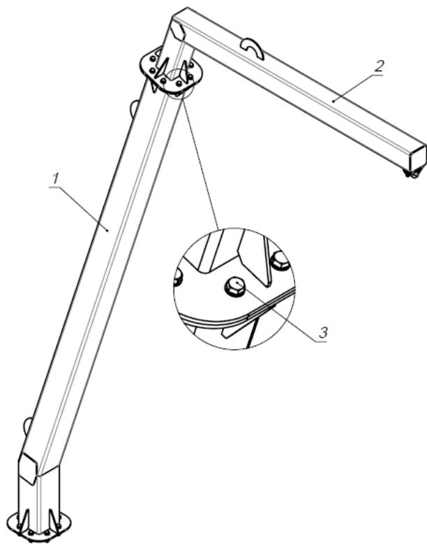
Рисунок 2 – Сборка верхней части стойки 1 – Стойка верх, 2 – Консоль, 3- Болтокомплект А
