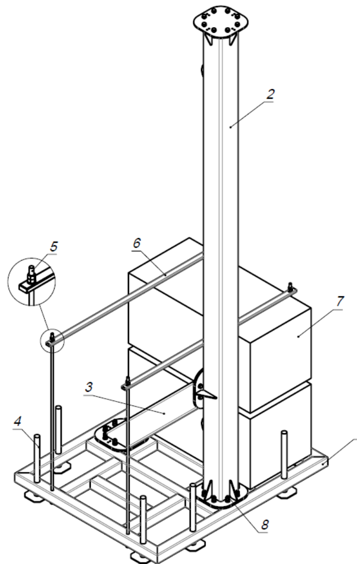
Рисунок 1 – Сборка основания.
