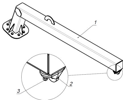
Рисунок 4 – Монтаж АУ «Дюраль»
