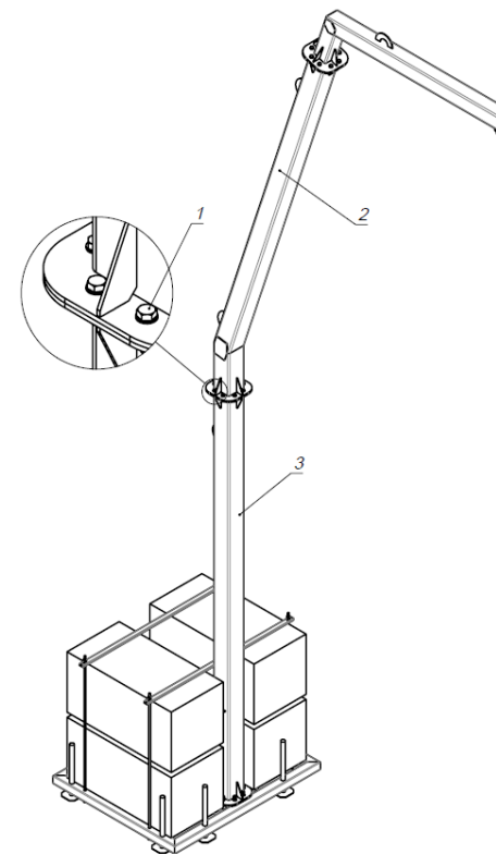
Рисунок 3 – Сборка стойки 1 – Болтокомплект А, 2 – Верхняя часть стойки, 3 – Нижняя часть стойки
