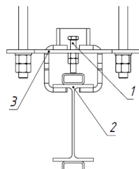
Рисунок 7 – Фиксация направляющих сегментов. 1 - Прижимной болт, 2 - Направляющий сегмент анкерной линии, 3 – Кронштейн универсальный с упором.
