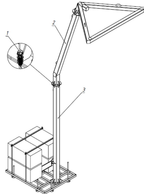
Рисунок 3 – Сборка стойки. 1 – Болтокомплект А, 2 – Верхняя часть стойки, 3 – Нижняя часть стойки
