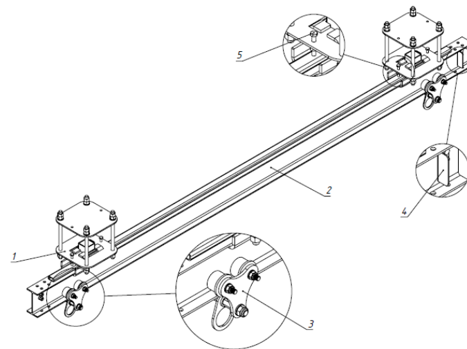
Рисунок 6 – Установка направляющих сегментов анкерной линии 1 – Кронштейн универсальный с упором, 2 – Направляющий сегмент анкерной линии, 3 – Мобильная анкерная точка, 4 – Концевой ограничитель, 5 – Прижимной болт.
