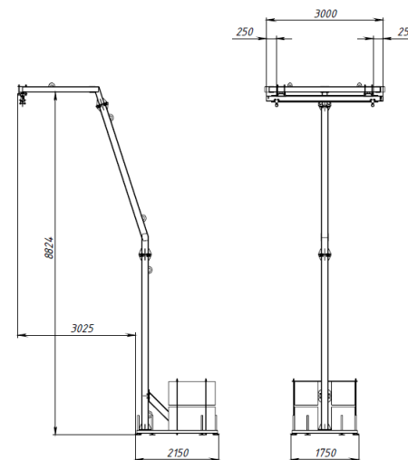
Рисунок 8 – Габаритные размеры системы
