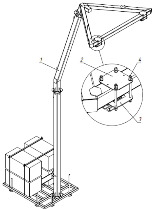
Рисунок 4 – Установка кронштейна на стойки. 1 – Стойка, 2 – Пластина, 3 – Кронштейн универсальный с упором, 4 – Шпилечный комплект Б;
