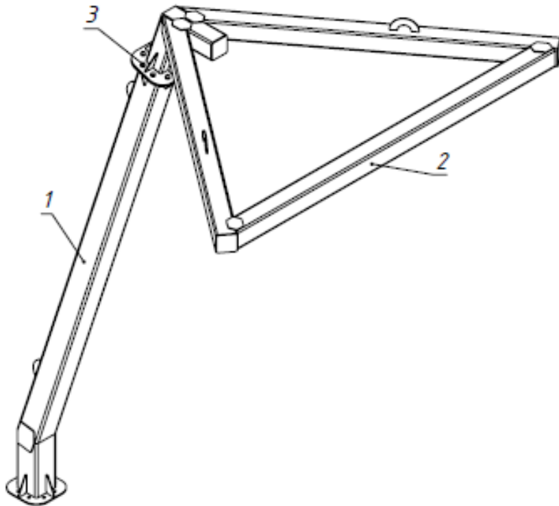
Рисунок 2 – Сборка верхней части стойки. 1 – Стойка верх, 2 – Консоль, 3- Болтокомплект А
