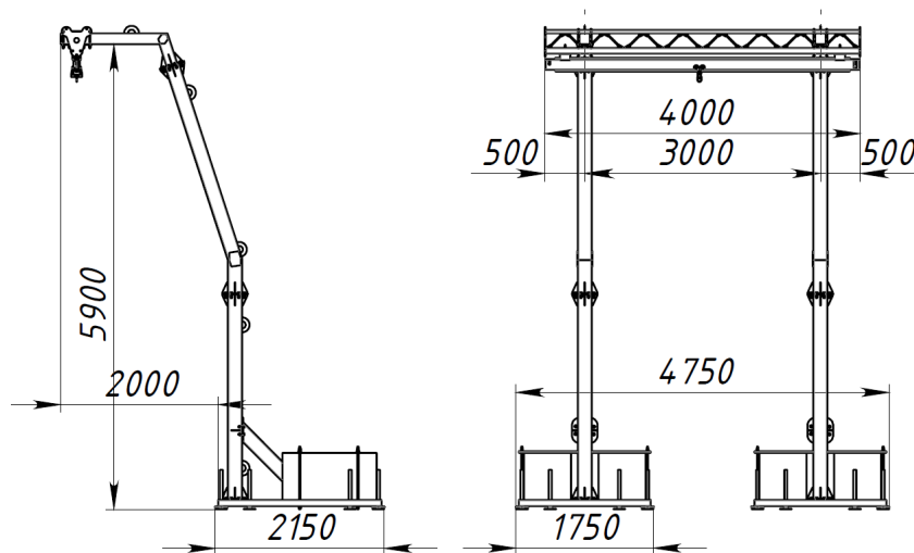
Рисунок 8 – Габаритные размеры системы
