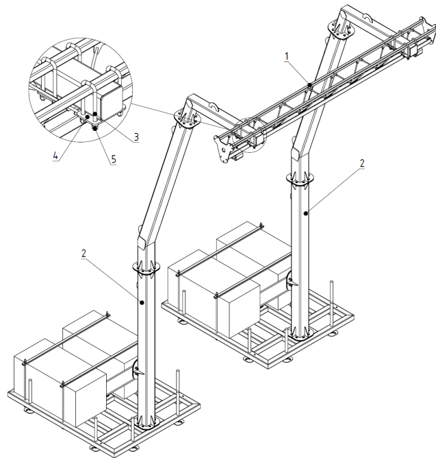
Рисунок 4 – Сборка фермы на стойки. 1 – Ферма пространственная 4м, 2 – Стойка, 3 – Скоба, 4 – Пластина, 5 – Болтокомплект В
