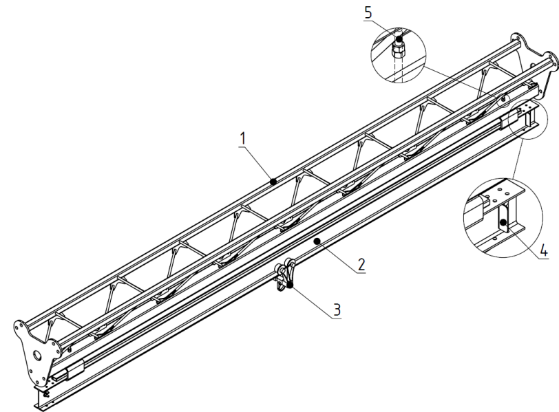
Рисунок 6 – Установка направляющих сегментов анкерной линии 1 – Пространственная ферма, 2 – Направляющий сегмент анкерной линии, 3 – Мобильная анкерная точка, 4 – Концевой ограничитель, 5 – Шпилечный комплект Б
