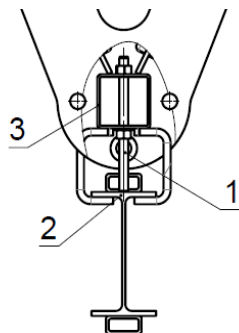
Рисунок 7 – Фиксация направляющих сегментов. 1 - Шпилечный комплект Б, 2 - Направляющий сегмент анкерной линии, 3 – Ферма пространственная
