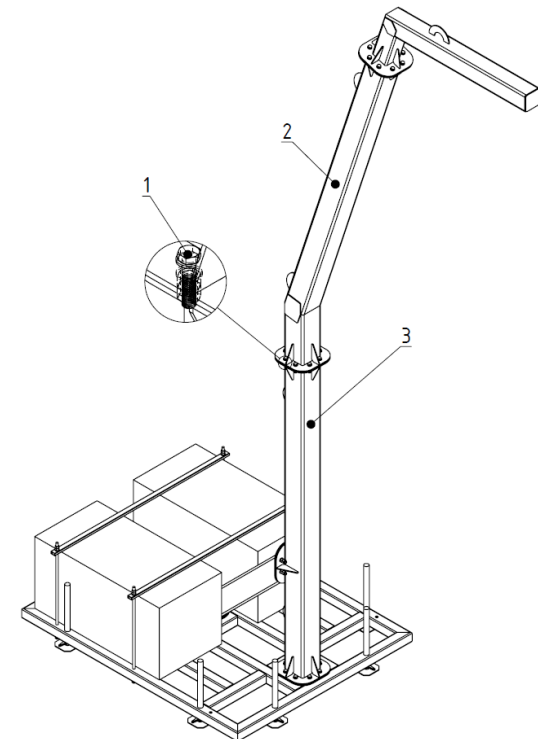
Рисунок 3 – Сборка стоек. 1 – Болтокомплект А, 2 – Верхняя часть стойки, 3 – Нижняя часть стойки
