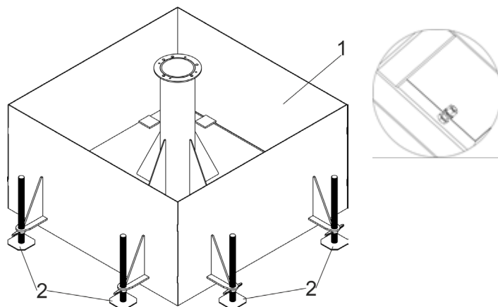
Рисунок 2. 1-Основание; 2-Аутригер.
