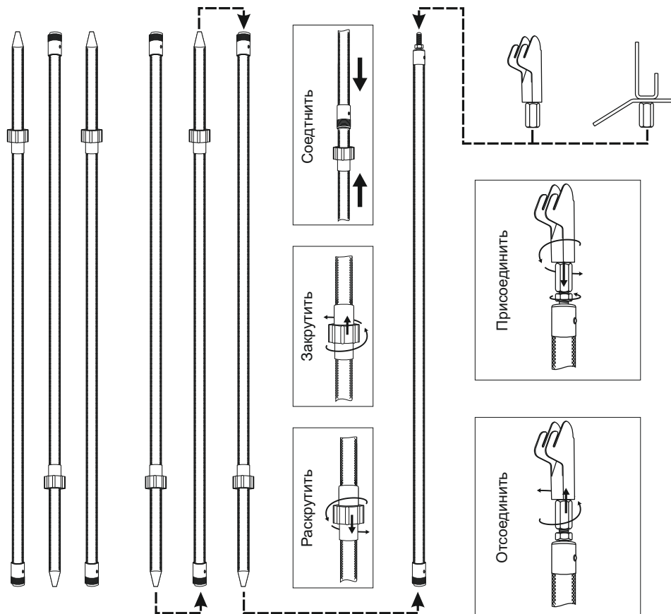
Рис. 2. Сборка
