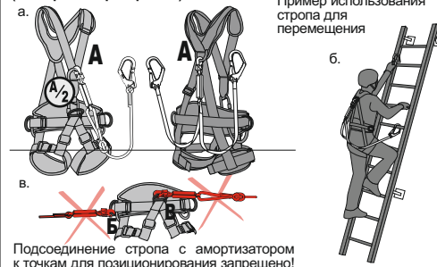
Рис. 5. Использование страховочного стропа (с амортизатором рывка)
