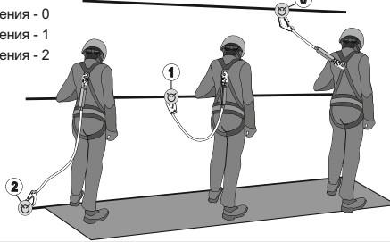
Рис. 5. Использование страховочного стропа (с амортизатором рывка)
