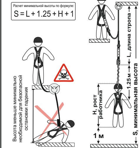
Рис. 8. Расчет высоты свободного пространства под пользователем для безопасной остановки падения
