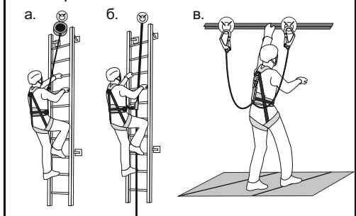
Рис. 9. Страховочная система
