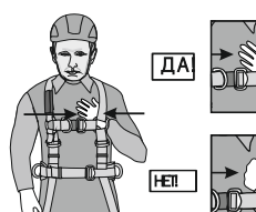
Рис. 8. Натяжение лямок
