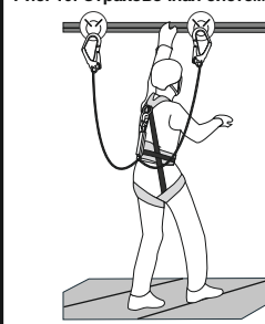
Рис. 10. Страховочная система
