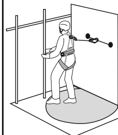
Рис. 11. Способ организации удерживающей системы
