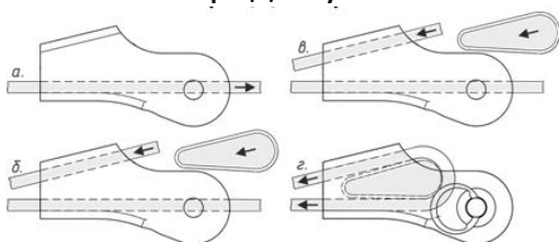
Рис. 3 Монтаж клинового зажима
