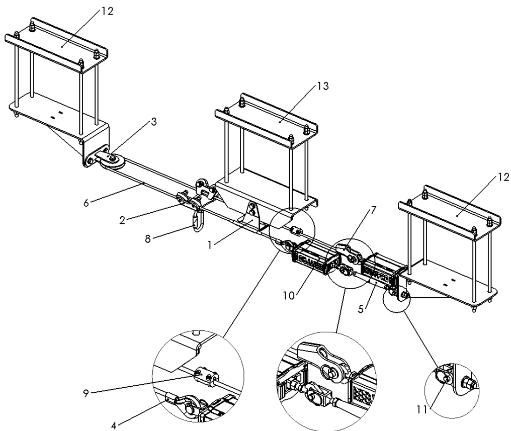
Рис.2 Монтаж анкерной линии
