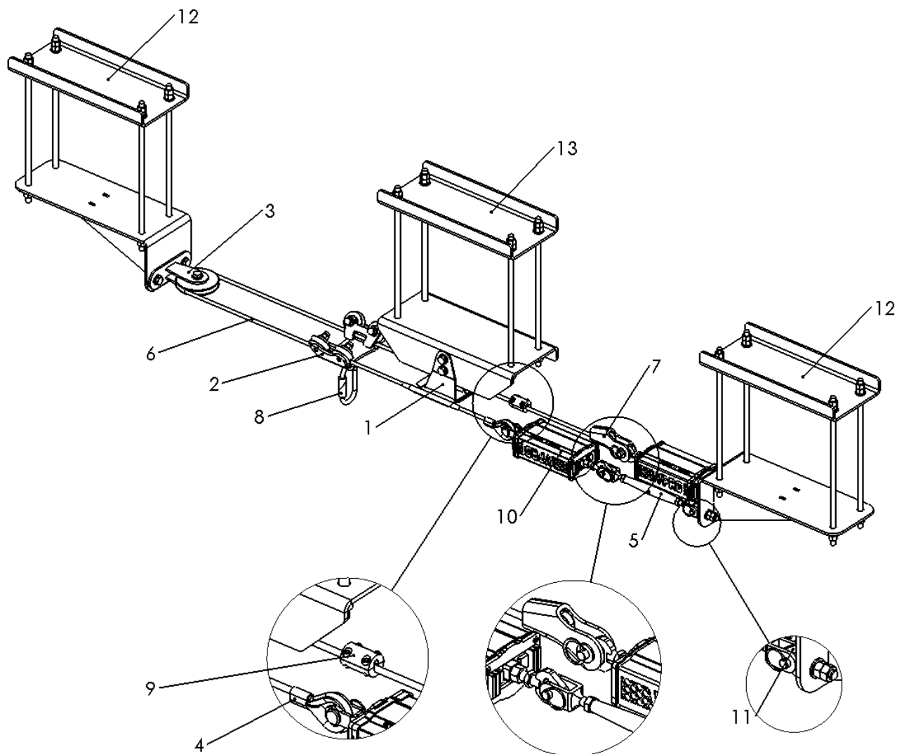
Рис.1 Основные составляющие анкерной линии «ТАНДЕМ»
