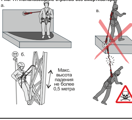
Рис. 11. Использование стропов без амортизатора
