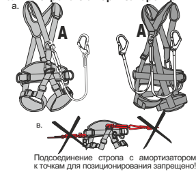
Рис. 5. В страховочных системах допускается использование только стропы с амортизатором рыка
