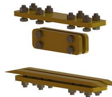
vpro DL L01/L02/H02 три комплекта элементов для соединения между собой сегментов анкерной системы в единое целое. Вместе образуют единый комплект - vpro DL L
