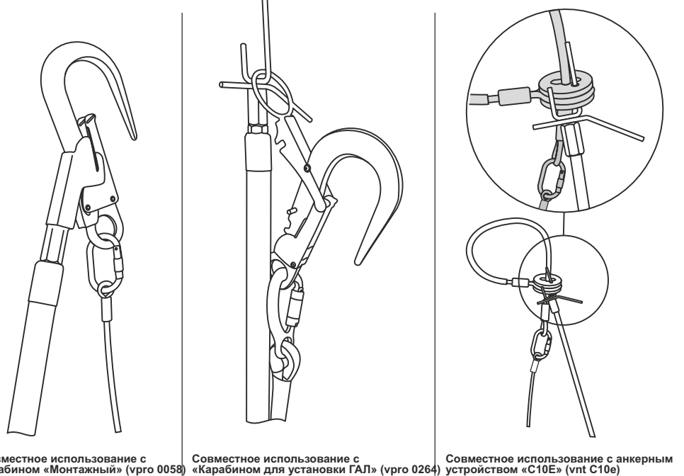
Рис. 3. Примеры использования наконечников с различными анкерными устройствами
