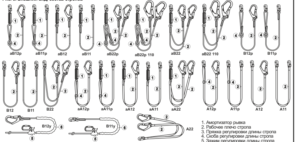
Рис. 3. Внешний вид, состав стропов
