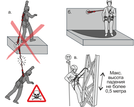
Рис. 9. Использование стропов без амортизатора.
